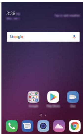
Home (default)
