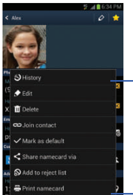
Sub-Menu items
